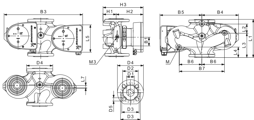
Рис. 33 Габаритные размеры, двоянные насосы, фланцевая версия со штекером
