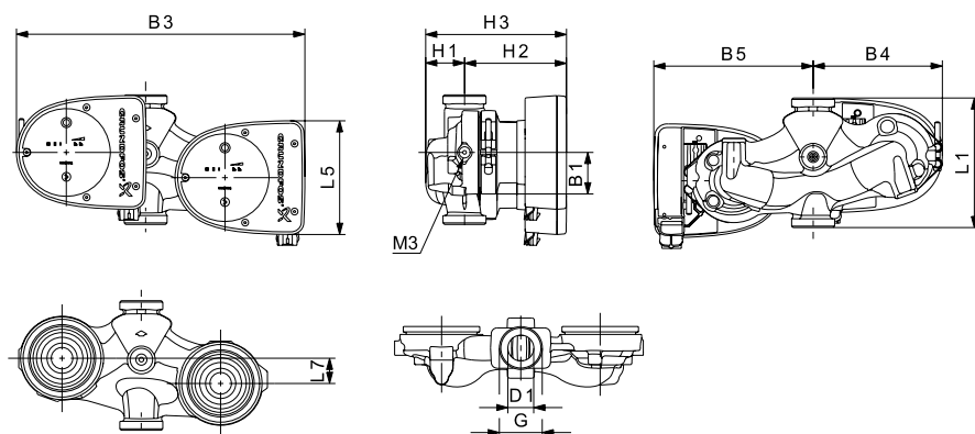
Рис. 30 Габаритные размеры, двойные насосы, резьбовая версия
